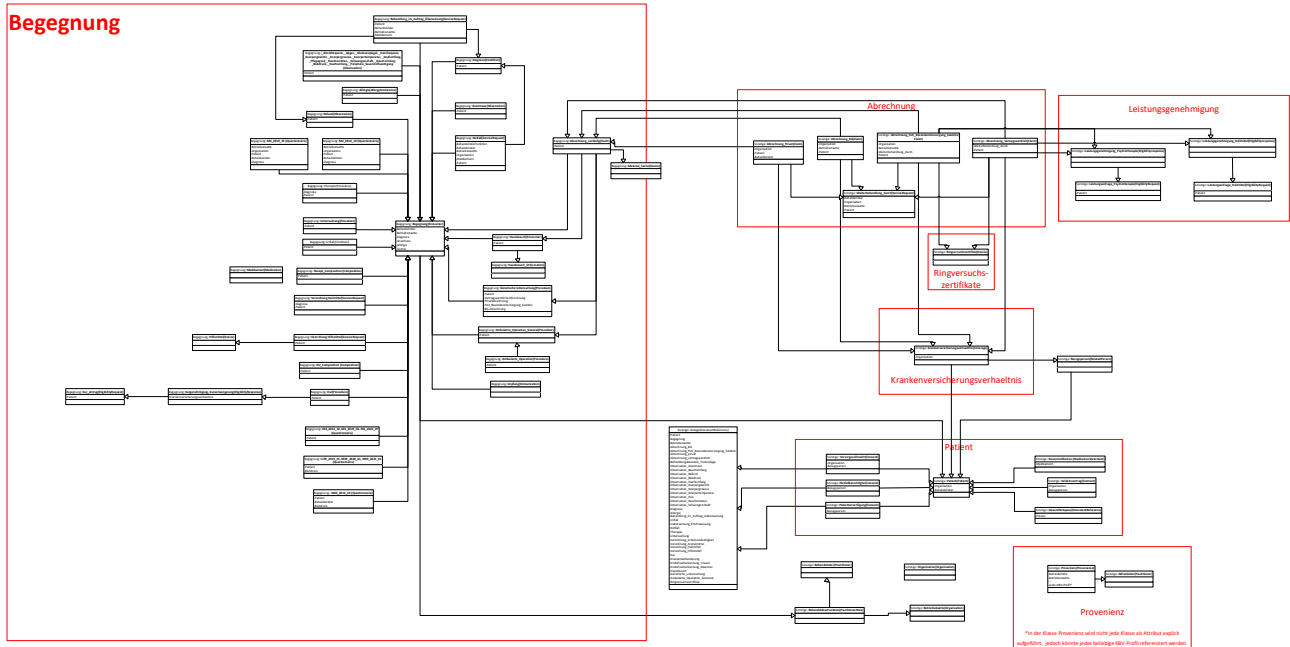
Abbildung 3 Ebene 1 des FHIR®-Informationsmodells
