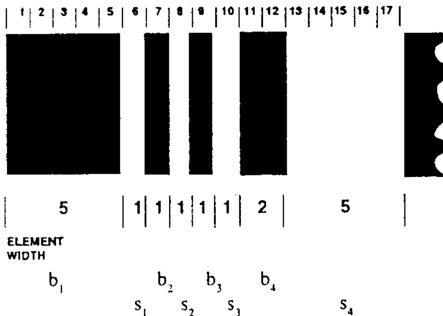
Abbildung 3: Codeword-Symbol
